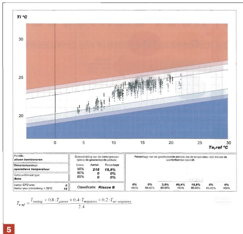
5 Grafische weergave van de adaptieve temperatuurgrenzen (ATG) voor een bèta-type gebouw
