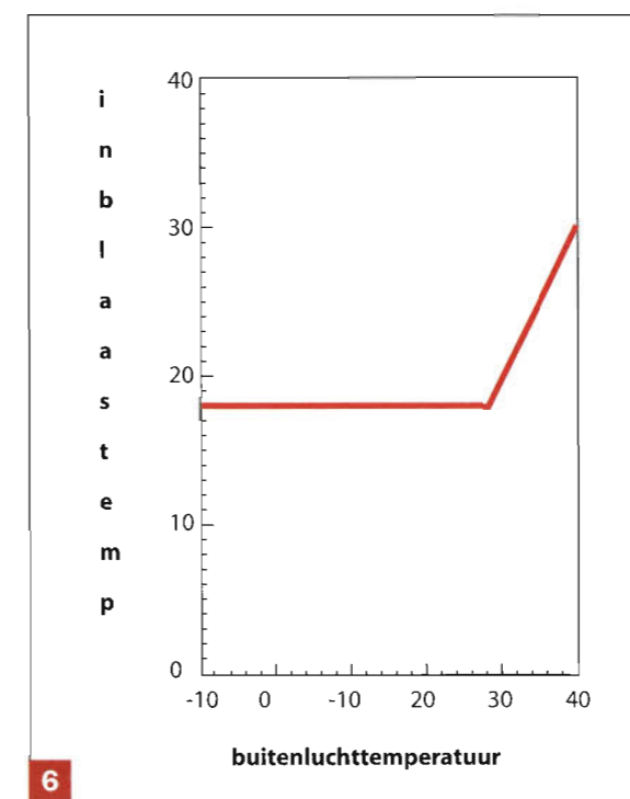
6 De relatie tussen buitenluchttemperatuur en inblaasttemperatuur bij topkoeling
