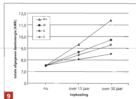
9 Topkoelingsconcept: totale afgegeven koelenergie, NEN 5060:2008 klimaatbestand voor energieberekeningen, KNMI klimaatscenario's na 15 en na 30 jaar
