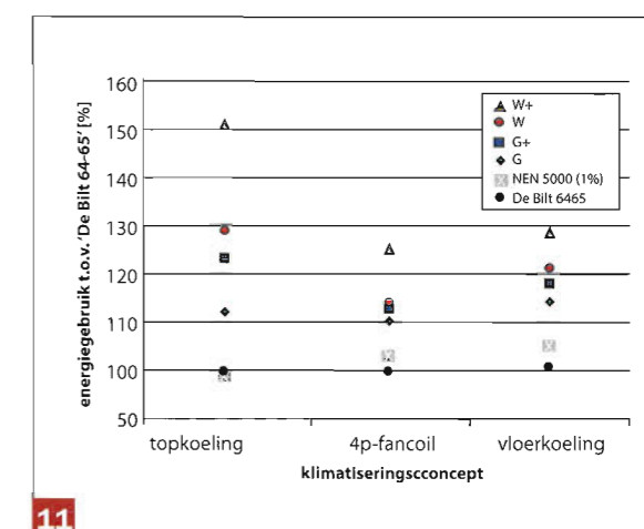
11 Vergelijking van 3 klimatiseringsconcepten: totale afgegeven koelenergie, NEN 5060:2008 klimaatbestand voor energieberekeningen, KNMI klimaatscenario's na 30 jaar, referentie: 'De Bilt 64-65'
