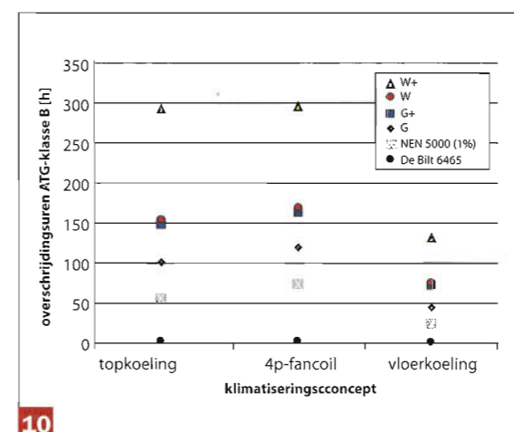
10 Vergelijking van 3 klimatiseringsconcepten: overschrijdingsuren van ATG-klasse B, NEN 5060:2008 klimaatbestand voor comfortberekeningen met 1% over-/ onderschrijdingskans, KNMI klimaatscenario's na 30 jaar, referentie: 'De Bilt 64-65'
